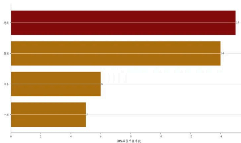
图 8 德国、日本、中国等国家高份额平台维持时长对比
